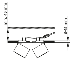
Strahler · Spot ↔ 18 x 8,7 cm, ↓ 12 cm excl. 2 x GU10, max. 35 W
