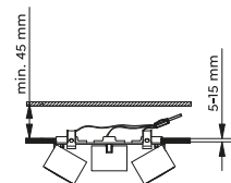
Strahler · Spot ↔ 27,3 x 8,7 cm, ↓ 12 cm excl. 3 x GU10, max. 35 W
